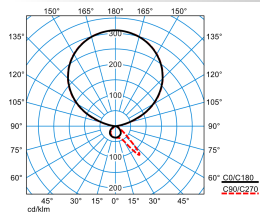
Luceos S BS G3 PAW-IL 125-830 ETDS KL 03
