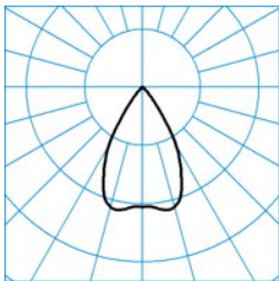
SNS RC5-HR1VFL-20-840
