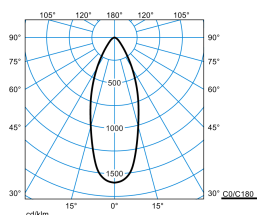
Amatris RC1 SRRFL 4/8/ML-9MC ET 05 + PC IP54 (stage 3)
