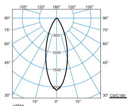
Amatris RC1 SRRFL 4/8/ML-9MC ET 05 + HC-19 05 (stage 5)
