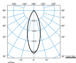
Amatris RC1 SRRFL 4/8/ML-9MC ET 05 + HC-19 05 (stage 3)
