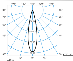
E-Line PRO 78 Lentyp L-SP 35-BF M54 ET 03 03
