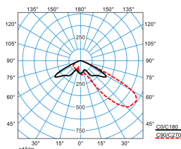
LnPlus 70-AM19L-SLR1/68000-730 56G1 ET (CLO initial value) TX390194
