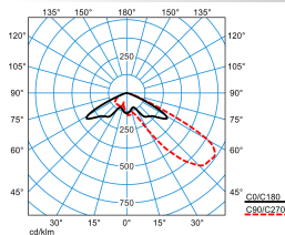
LnPlus 70-AM19L-SLR1/68000-730 56G1 ET (CLO end value) TX390090
