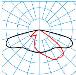
LnPlus 60-AB7L-LR/32000-740 24G1 ET (CLO end value) TX377703 ■ C0 - C180 ■ C90 - C270 DIN 5040: A30 UTE: 1,00 E DLOR: 100 % ULOR: 0 % CEN Flux Code: 39 76 98 100 100
