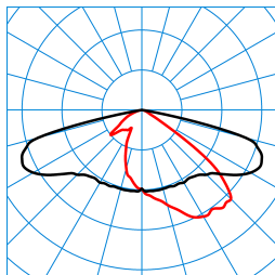
LnPlus 60-AB7L-LR/32000-740 24G1 ET (CLO initial value) TX377234 ■ C0 - C180 ■ C90 - C270 DIN 5040: A30 UTE: 1,00 E DLOR: 100 % ULOR: 0 % CEN Flux Code: 39 76 98 100 100
