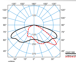
LnPlus 40-AB7L-SLR1/5100-727 6G1 ET (CLO initial value)
