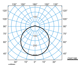
Olisq RWD2 DW 20-840 ETBLE +CAS IP54 + Olisq RWD2 ZDR 1/2 03
