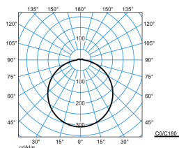
Olisq RWD2 DW 20-840 ETBLE +CAS IP54 + Olisq RWD2 C 01
