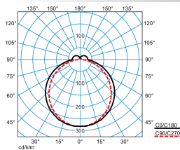
Olisq LWD1 DW 40-8TW ETDD8 IP54 IK (DWW)
