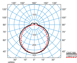
Olisq LWD1 DW 40-8TW ETDD8 IP54 IK (DCW)
