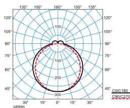
Olisq LWD1 DW 40-8TW ETDD8 IP54 IK (DSU)
