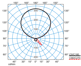
Luceos S-T G3 PAW-IL 300-830 ETDS 03 (LEO1)
