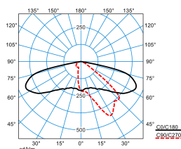
Publisca P3-AB2L-LR/5100-740 6G1 ET (CLO initial value)
