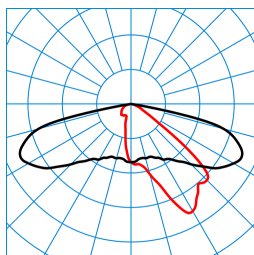
Publisca P3-AB2L-LR/5100-740 6G1 ET (CLO initial value) TX301626
