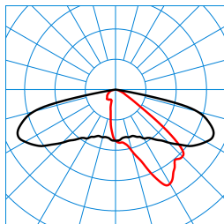
Publisca P3-AB2L-LR/5100-740 6G1 ET (CLO end value) TX301930
