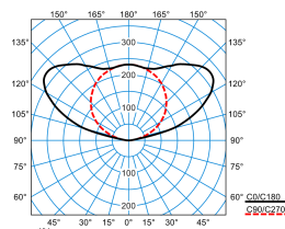
E-Line PRO 78HE I-UW 30-840ET L75 01 01
