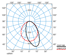
SFlow D2-L MLA LED4600-830 ETDD 01 TX770171
