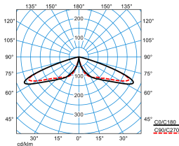
CS 19 100-RB6L-LR/1800-740 2G1S ET (CLO end value)
