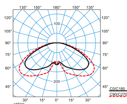
Publisca P1W-RBT-LRA/3200-730 4G1S ET (CLO initial value)
