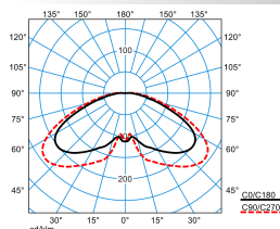
Publisca P1W-RBT-LRA/3200-730 4G1S
