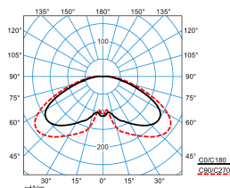
Publisca P1W-RBT-LRA/3200-730 4G1S ET (CLO end value)
