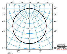
Olisq QWD2 DW 20-840 ETBLE +DMR IP54 + Olisq QWD2 ZDR 1/1 01
