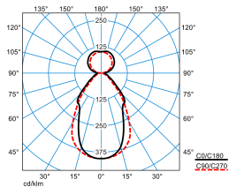
SFlow H2-L CDP-I 6300-830 ET 03
