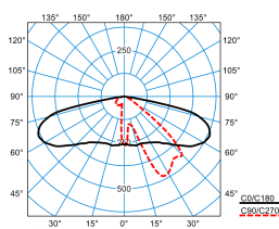
Publisca P1-AB2L-LRA/1000-740 2G1S ET (CLO initial value) TX301046 DIN 5040: A30 UTE: 1,00 G DLOR: 100 % ULOR: 0 % CEN Flux Code: 34 70 96 100 100
