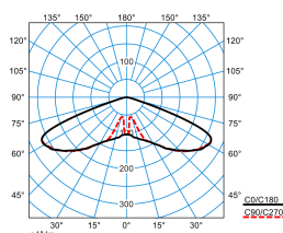
Publisca P2-RB6L-LR/1200-730 2G1S ET (CLO end value)
