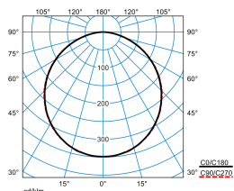
Olisq QWD3 DW 30-830 ETBLE +DMM IK + Olisq QWD3 ZDR 1/1 05
