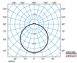
Olisq QWD3 DW 30-830 ETBLE +DMM IK
