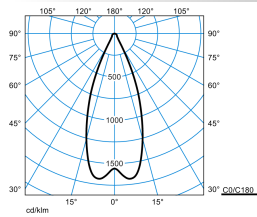
Lim 3P RF-FL 40-EW M50 ETDD L1,5 05
