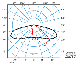
LIQ 50N-AB2L-LR/2000-740 2G1 ET (CLO initial value) TX777488
