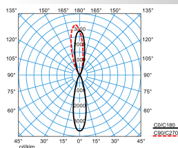
OsidoRW-RE3L/RE3L-10-830-ET-GS26
