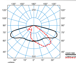
LIQ 70N-AB7L-LRA/6800-730 8G1 ETDD(CLO end value) TX277910
