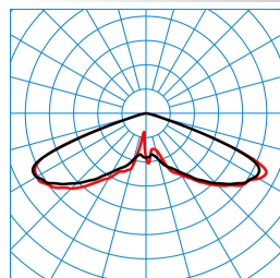
Publisca P2-RB6L/2000-740 3G1S TX047820 ■ C0 - C180 ■ C90 - C270 DIN 5040: A20 UTE: 1,00 J DLOR: 100 % ULOR: 0 % CEN Flux Code: 20 57 98 100 100
