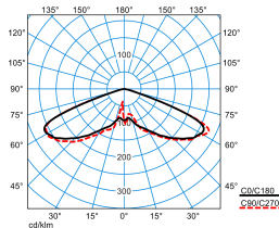
Publisca P2-RB6L/2000-740 3G1S TX047820 DIN 5040: A20 UTE: 1,00 J DLOR: 100 % ULOR: 0 % CEN Flux Code: 20 57 98 100 100
