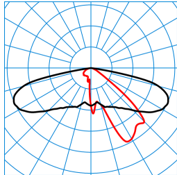
Publisca P1-AB2L-LR/2600-740 3G1S TX047524 ■ C0 - C180 ■ C90 - C270 DIN 5040: A30 UTE: 1,00 l DLOR: 100 % ULOR: 0 % CEN Flux Code: 34 71 96 100 100
