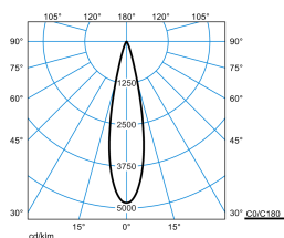
7651 Lentyp L-SP 40-EC M39 ET 03 (225)
