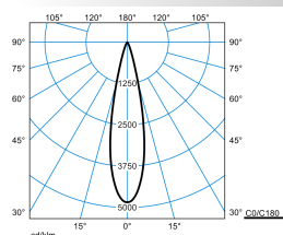
7651 LentyP L-SP 40-EC M39 ET 03 (150)
