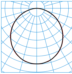
Olisq QWD2 DW 35-840 ETBLE +DMR IP54 IK + Olisq QWD2 ZDR 1/1 03 TX461490
