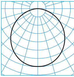
Olisq RWD3 DW 50-830 ET PC + Olisq RWD3 ZDR 1/1 01 TX426603
