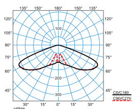
Publisca P1-RB6L-LR/1100-730 2G1S ET (CLO end value)
