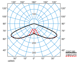
Publisca P1-RB6L-LR/1100-730 2G1S
