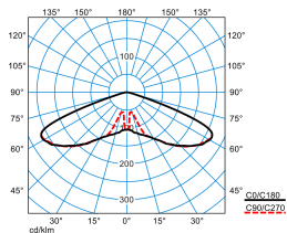
Publisca P1-RB6L-LR/1100-730 2G1S ET (CLO initial value)
