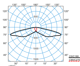
Publisca P3-SB3L-SLR1/2200-740 2G1
