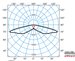
Publisca P3-SB3L-SLR1/2200-740 2G1 ET (CLO end value)
