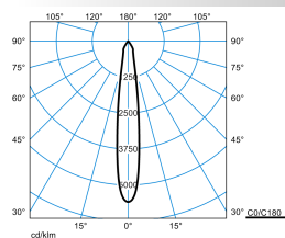
E-Line PRO 78 BV G2 RF-SP 50-840 M35 ETDD 05 Blank
