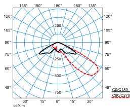
LnPlus 60-AM19L-SLR2/24000-722 18G1 ET (CLO end value)
