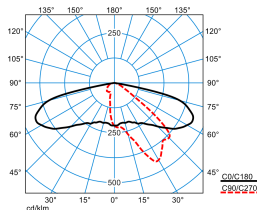
Cuvia 60-AB2L-LRA/7500-740 12G1S ET
