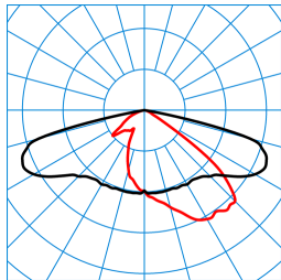
LIQ 70N-AB7L-LR/8200-740 10G1 ET(CLO end value) TX277872 ■ C0 - C180 ■ C90 - C270 DIN 5040: A30 UTE: 1,00 E DLOR: 100 % ULOR: 0 % CEN Flux Code: 39 76 98 100 100
