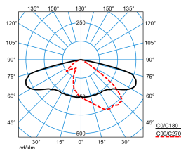
LIQ 70N-AB7L-SLR2/13000-722 12G1 ET (CLO end value)
