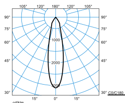
E-Line PRO 78 BV G2 RF-MF 40-840 M35 ET 01 01
