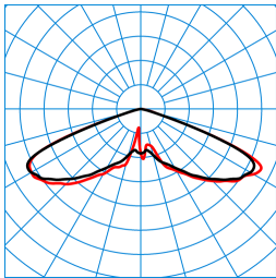
Publisca P2-RB6L/2000-730 3G1S TX047819 ■ C0 - C180 ■ C90 - C270 DIN 5040: A20 UTE: 1,00 J DLOR: 100 % ULOR: 0 % CEN Flux Code: 20 57 98 100 100
