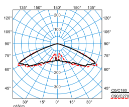
Publisca P1W-RB6L-LRA/1200-730 2G1S ET (CLO initial value)
