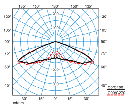
Publisca P1W-RB6L-LRA/1200-730 2G1S ET (CLO end value)
