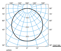
Olisq RWD3 DW 30-840 ETDD IP54 PC + Olisq RWD3 ZDR 1/1 01
