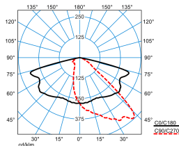
Cuvia 60-AB6L-LRA/5100-740 8G1S ET
