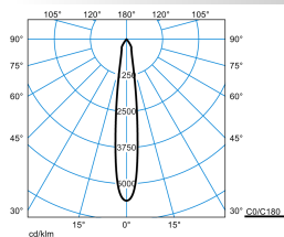
E-Line PRO 78 BV G2 RF-SP 20-835 M34 ET 01 Blank
