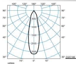
TaroMini 3PTD RF-MF 40-830 M33 ET 01
