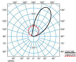
Altigo G2 60 WO GS AM15L/350-830 + VE IP66 24V DC 80W
