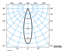
E-Line PRO 78 Lentyp L-MF 35-BF M54 ET 05 Blank
