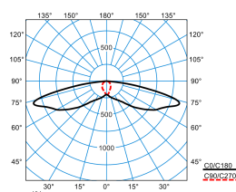
LIQ 50N-SB3L-LR/1350-727 2G1 ET (CLO end value)
