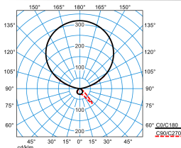
Luceos S G3 PAW-IL 170-8TW ETDS FT 01 (DWW)
