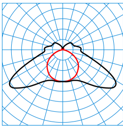
Tugra 15 PXW 50-840 ET IP69K 23 TX303027
