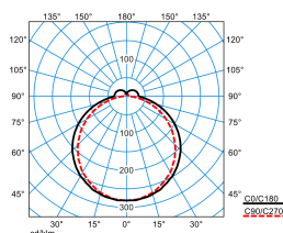
Olisq LWD2 DW 20-60/4/ML-830 ET IK (stage 2)
