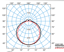
Olisq LWD2 DW 20-60/4/ML-830 ET IK (stage 1)
