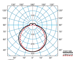
Olisq LWD2 DW 20-60/4/ML-830 ET IK (stage 4)
