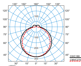
Olisq LWD2 DW 20-60/4/ML-830 ET IK (stage 3)
