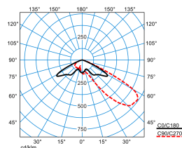
LnPlus 40-AM19L-SLR3/10000-722 8G1 ET (CLO end value)
